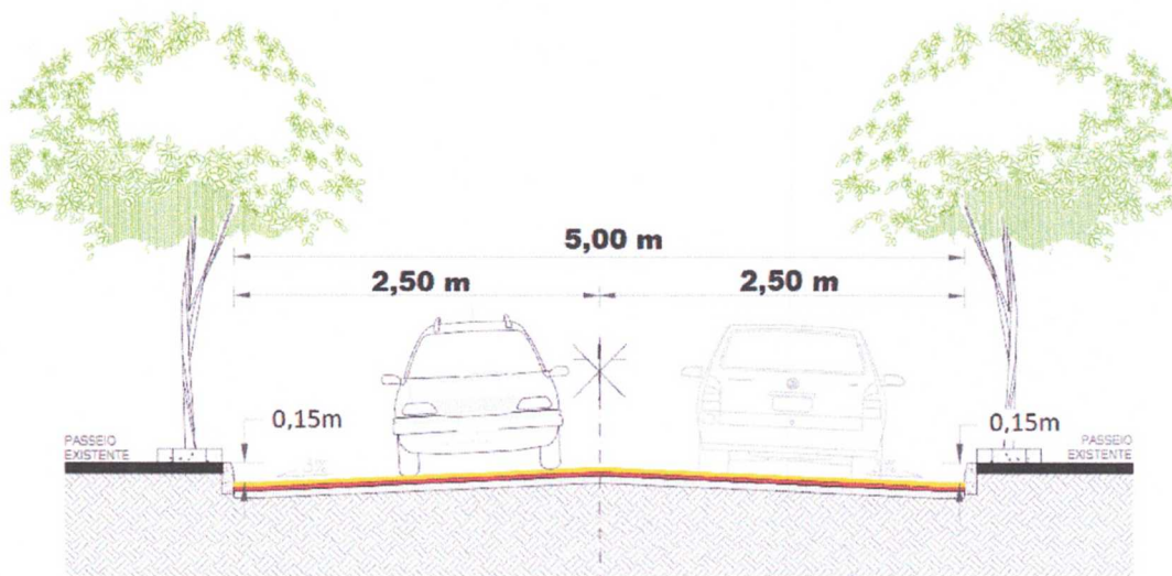
SEÇÃO TIPO DE PAVIMENTAÇÃO
