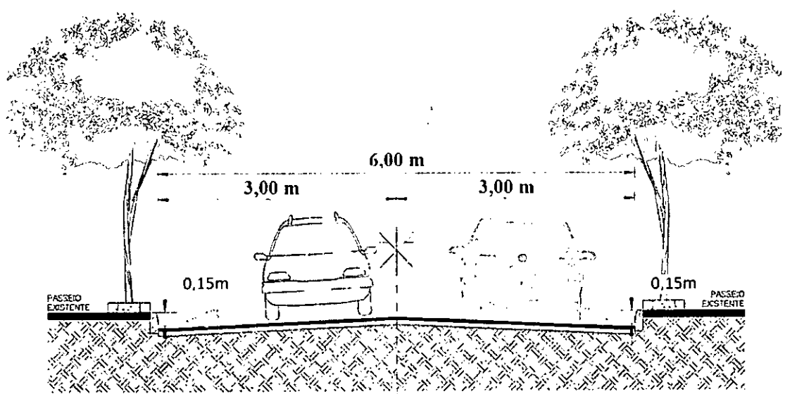
SEÇÃO TIPO DE PAVIMENTAÇÃO
