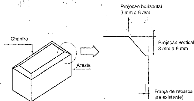
Figura 1 – Chanfro de uma peça de concreto
