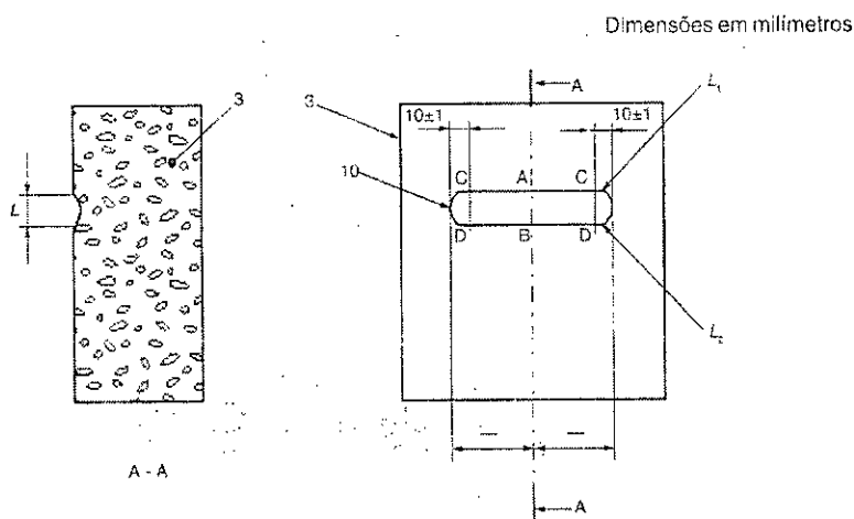
Figura C.2 — Medição da cavidade na amostra ensaiada
